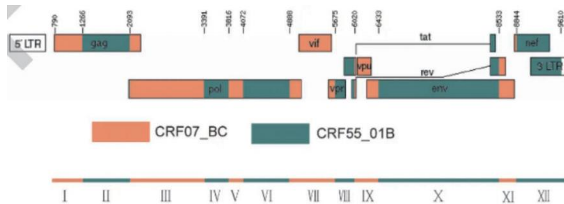
HIV-1CRF172_0755近全长基因组
